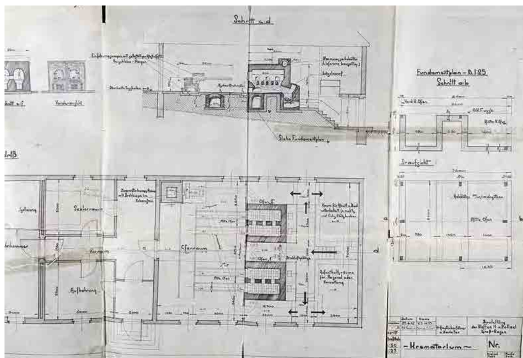
Чертеж крематориев, построенных фирмой «Топф» в концентрационных лагерях Освенцим и Гросс-Розен. 25 июня 1942 г. Фрагмент. ЦА ФСБ России. АУД № Н-19262. Л. 381.
